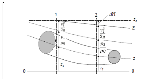
Slika7. Grafički prikaz Bernoullijeve jednadžbe za realne tekućine, [5]
