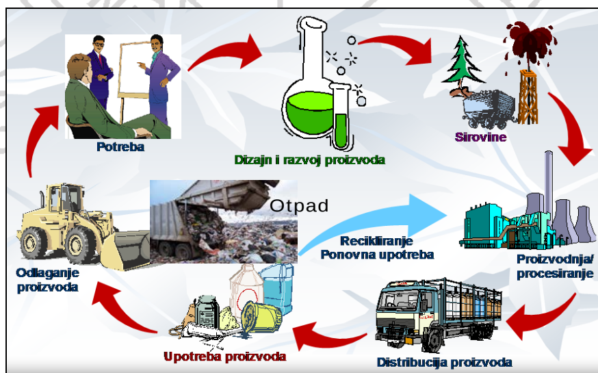
Slika 5. Industrijska simbioza održivosti u proizvodnji/primeni pesticida
